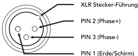
Abb. 5 – XLR-Anschluss
