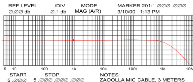
Abb.: Frequenzgang des Zaolla Silverline Mikrofonkabels, Länge 3m
