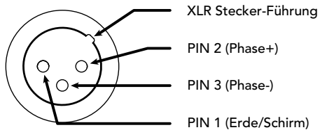
Abb. 2 – XLR-Anschluss
